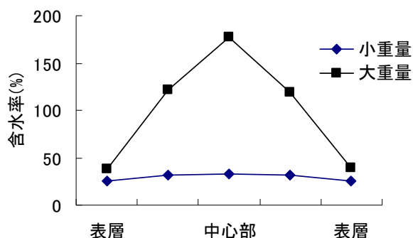
図-2 水分傾斜
